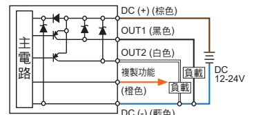
EP45□ - 04 - □ 2PNP + 複製功能
