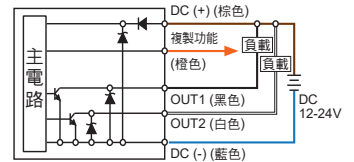
EP45□ - 02 - □ 2NPN + 複製功能
