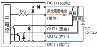
EP45□ - 030 - □ 2PNP + Analog 輸出 (1 ~ 5 V)
