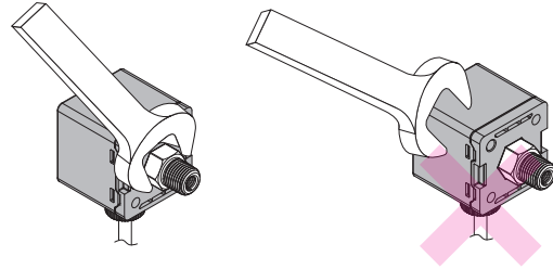
EP45□ - 02 - □ 2NPN + 複製功能
